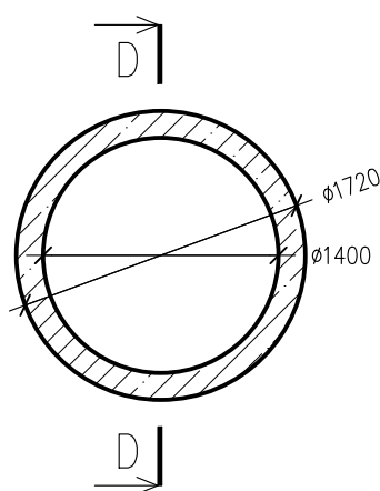
PRZEKRÓJ C-C
